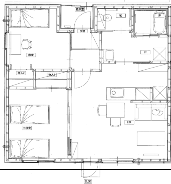
2LDK間取り図 63.35㎡ (参考)
